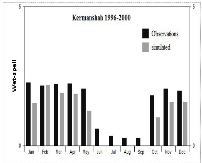
شکل ۲- صحت سنجی مدل SDSM نسبت به بارش
