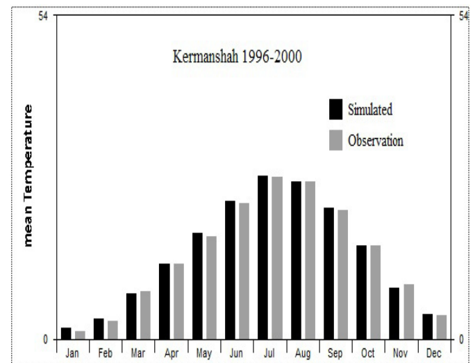
شکل ۳- صحت سنجی مدل SDSM نسبت به دما
