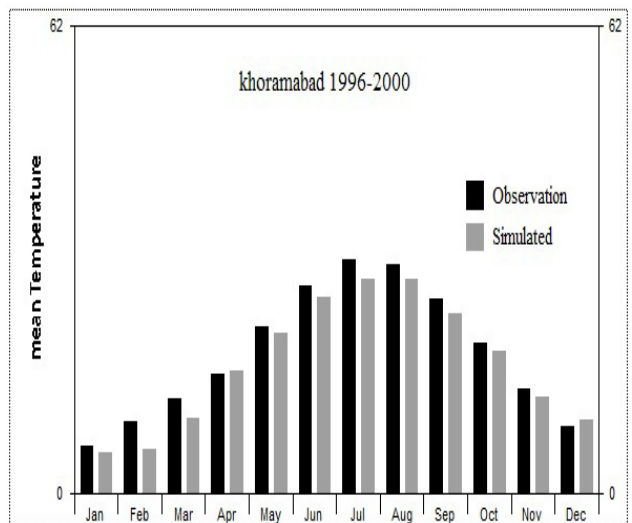
شکل ۳- صحت سنجی مدل SDSM نسبت به دما
