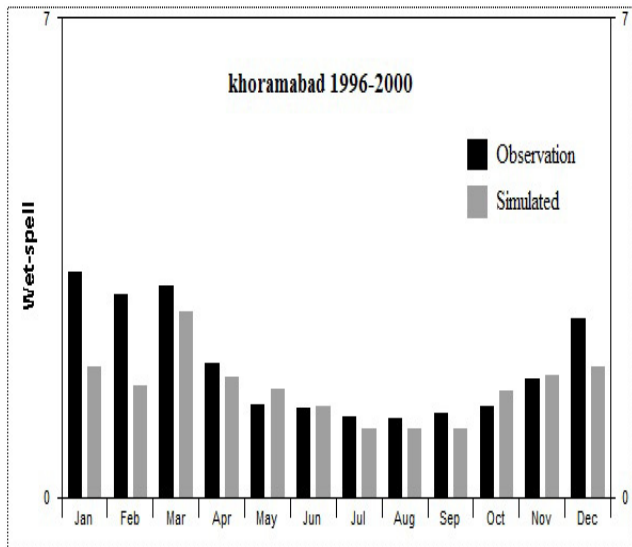
شکل ۲- صحت سنجی مدل SDSM نسبت به بارش
