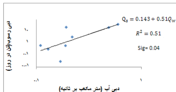
شکل ۴- منحنی سنج رسوب دوره خشکسالی در حوضه سنوبر
