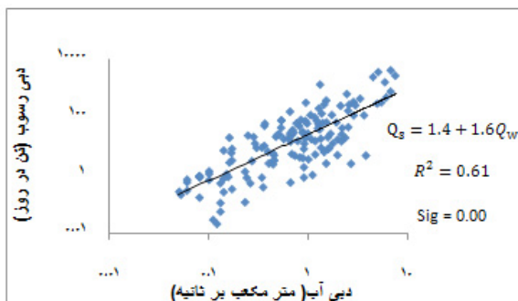
شکل ۳- منحنی سنج رسوب دوره نرمال در حوضه سنوبر
