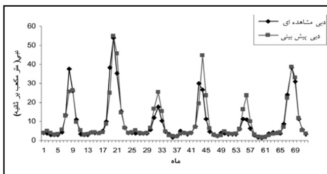
شکل ۸- مقادیر دبی مشاهده‌ای و پیش‌بینی شده با AMRA(3, 1)
