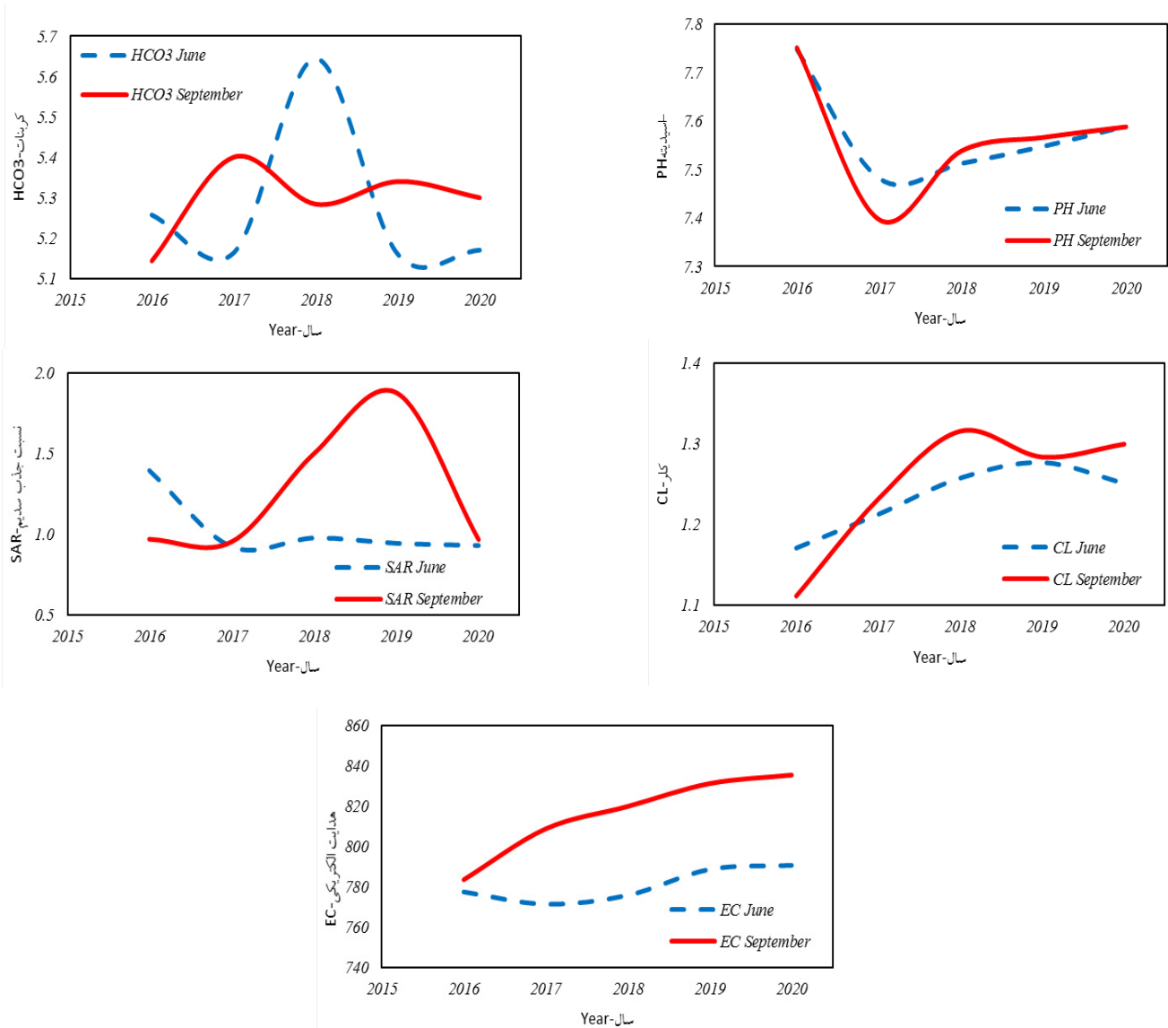
شکل ۳- تغییرات سالانه پارامتر \text{HCO}_3 ، PH (میلی اکی والان برلیتر)، CL (میلی اکی والان برلیتر)، SAR (میلی اکی والان برلیتر) و EC (میلی موس برمتر) در ماه‌های خرداد و شهریور
