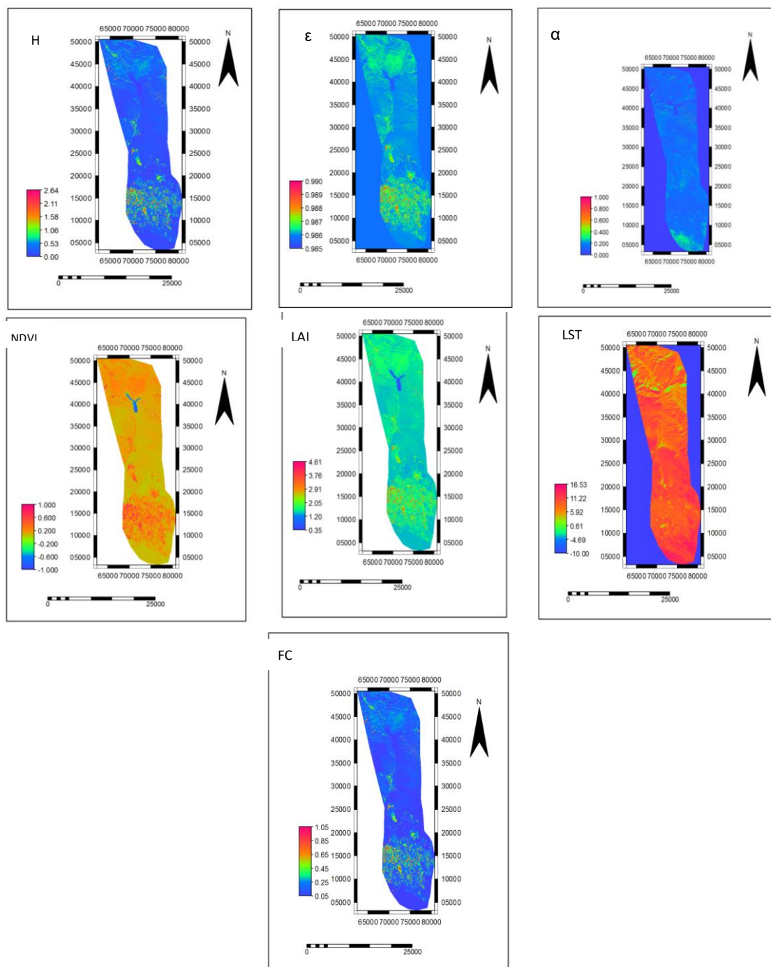
شکل ۳- تهیه لایه‌های ورودی مدل SEBS در ابتدای دوره رشد (۲۰۲۰/۱۲/۲۴) شامل (شار حرارتی محسوس H، گسیبندی \epsilon ، آلبیدو \alpha ، شاخص پوشش گیاهی NDVI، شاخص سطح برگ LAI، دمای سطح LST، درصد پوشش گیاهی FC)
