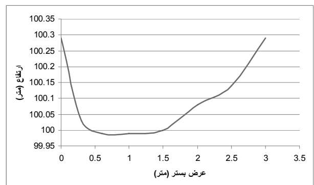
شکل ۷- اولین مقطع آبراهه زیرحوزه‌ی دارای عملیات آبخیزداری واقع در بالادست سازه‌ها
