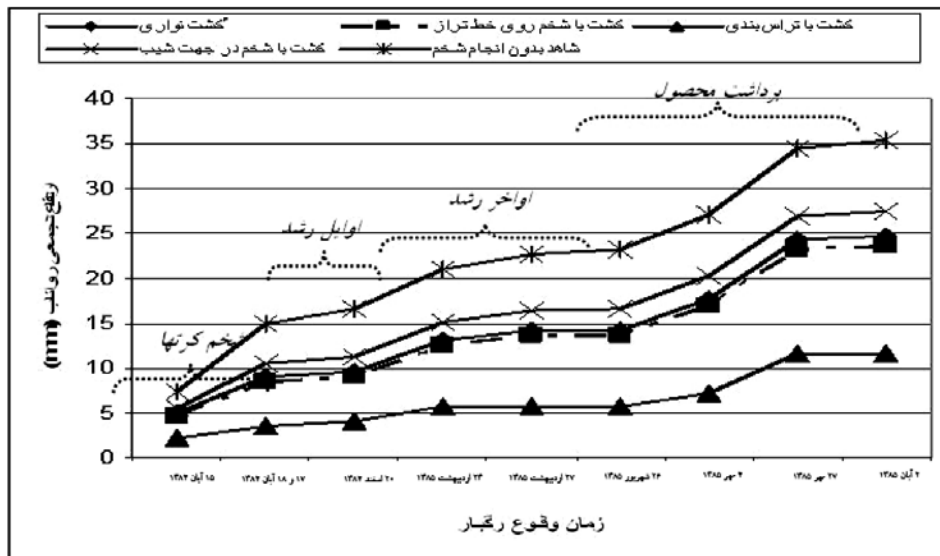
شکل ۵ - همزمانی مقادیر تجمعی رواناب و تقویم زراعی منطقه در سناریوهای مدیریتی مختلف
