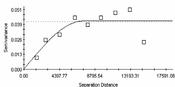
شکل ۱۱ - واریوگرام SAR
