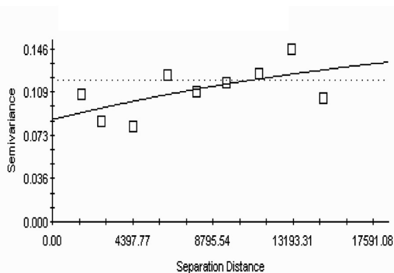
شکل ۳ - واریوگرام مجموع کاتیون‌ها
