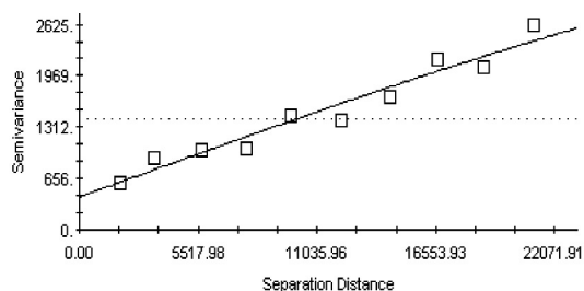
شکل ۱۰ - واریوگرام متقابل TH
