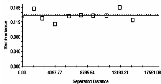
شکل ۹ - واریوگرام TH
