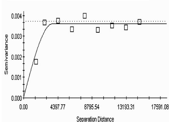
شکل ۵ - واریوگرام سدیم
