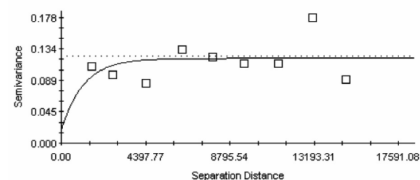
شکل ۱۳ - واریوگرام کلر
