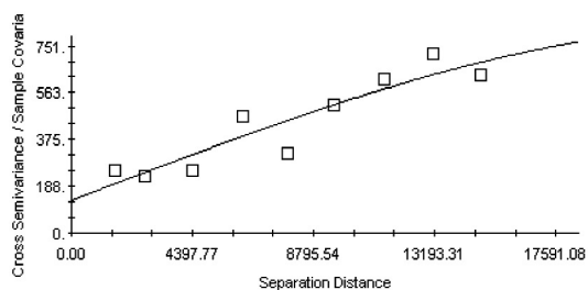
شکل ۱۲ - واریوگرام متقابل SAR
