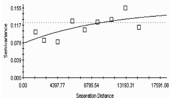
شکل ۷ - واریوگرام TDS
