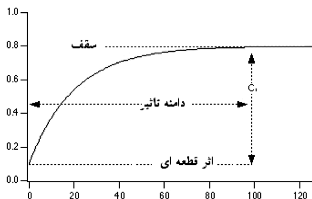
شکل ۲ - نمایی از یک واریوگرام
