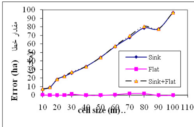
شکل ۷- خطای چاله و سطح صاف در DEM ۱/۲۵۰۰۰ Fig 7. Sink and flat error in Dem of 1/25000
