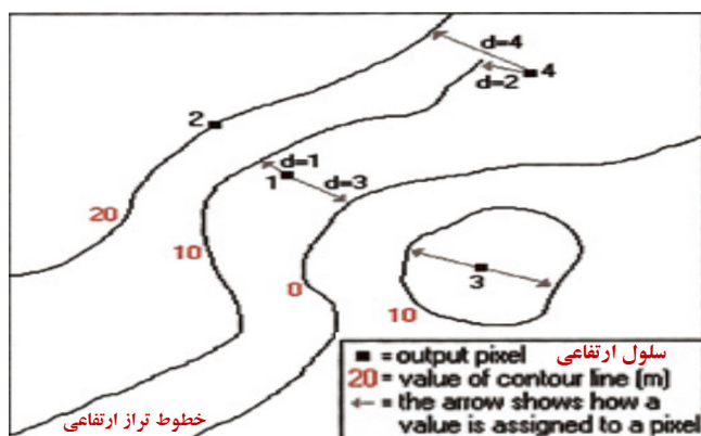
شکل ۹- الگوریتم درونیابی خطی.
