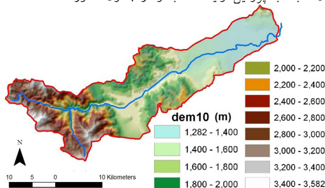
شکل ۸- نمایش مدل ارتفاع رقومی (DEM) حوزه آبخیز شهرچایی.
