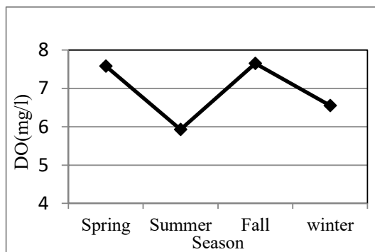
شکل ۴- تغییرات فصلی DO در رودخانه بابلرود (مشاهداتی)
