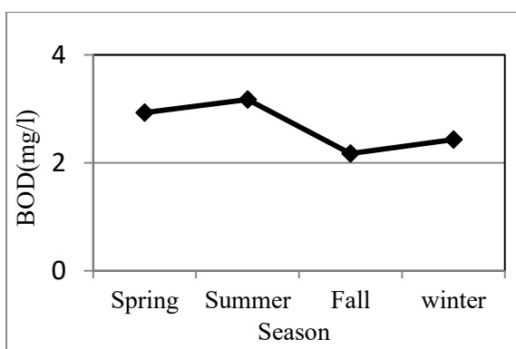
شکل ۵- تغییرات فصلی BOD در رودخانه بابلرود (مشاهداتی)
