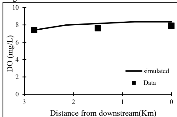
شکل ۱۱- شبیه سازی DO رودخانه بابلرود- آزمون پاییز ۹۷
