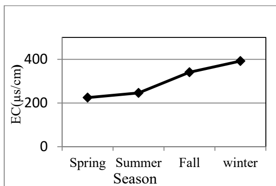
شکل ۶- تغییرات فصلی EC در رودخانه بابلرود (مشاهداتی)
