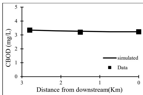
شکل ۱۰- شبیه سازی CBOD رودخانه بابلرود-آزمایش پاییز ۹۷
