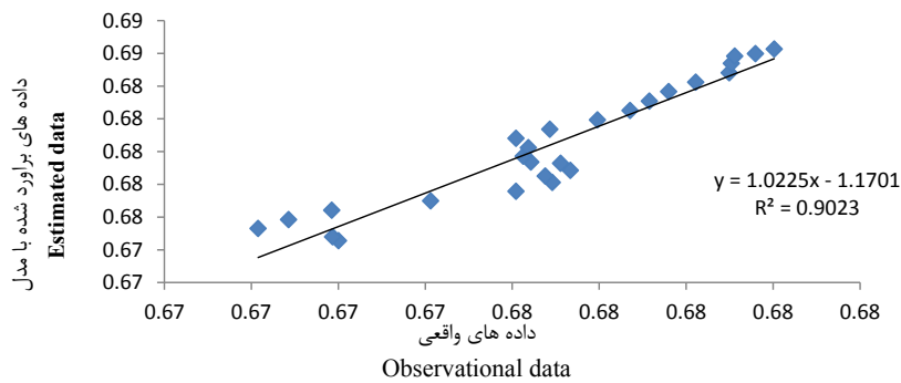
شکل ۵- نتایج حاصل از ارزیابی مدل HARTT با داده‌های اندازه‌گیری شده تراز آب زیرزمینی. Fig .5.The results of the evaluation HARTT model using observed data of ground water level.
