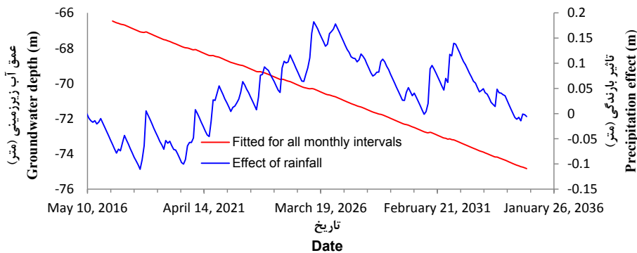
شکل ۶- تغییرات بارندگی موثر و نوسانات تراز آبخوان در سال‌های آینده. Fig .6.Changes in the effective rainfall and aquifer level fluctuations in the future.
