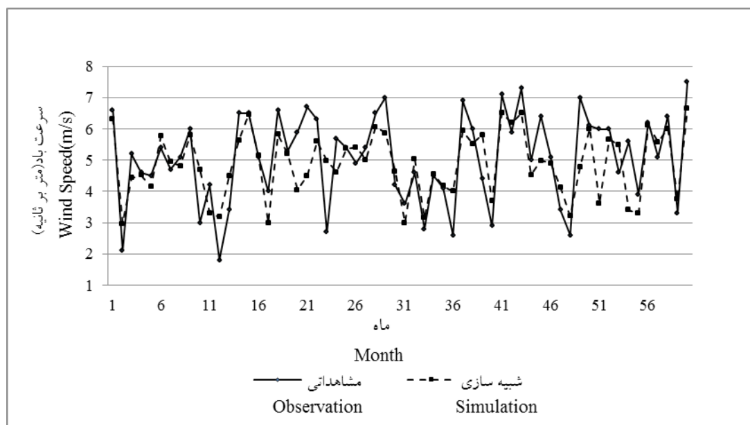
نمودار ۱- مقایسه مقادیر واقعی و پیش‌بینی شده سرعت باد در ترکیب دو شبکه‌های فازی-عصبی
