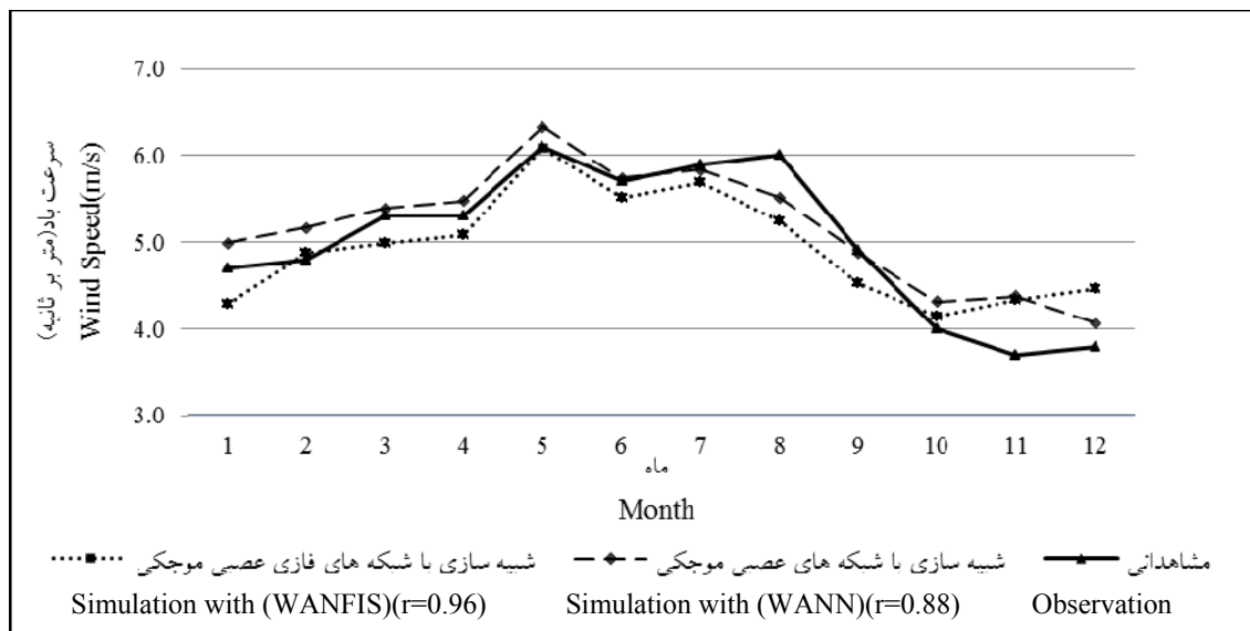
نمودار ۳- مقایسه مقادیر مشاهداتی و شبیه سازی شده با دو مدل عصبی موجکی و فازی-عصبی موجکی سال ۱۳۸۴
