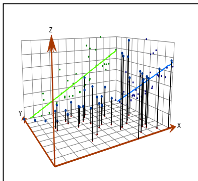
شکل ۱۰- تغییرات مکانی نهشته های کوآترنر ( Q_1 )
