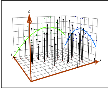
شکل ۹- تغییرات مکانی نهشته های کوآترنر ( Q_2 )
