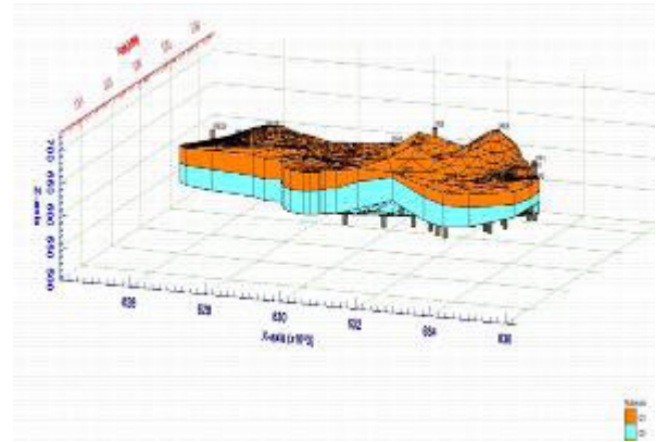
شکل ۷- بلوک دیگران نهشته های کوآترنر Q_1 ، چاه ها و سونداژهای ژئوالکتریک
