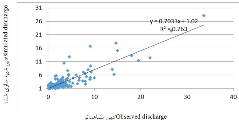
شکل ۳- نمودار همبستگی مقادیر دبی مشاهداتی و شبیه‌سازی شده دوره واسنجی ۱۳۸۵-۱۳۷۱ Fig 3. Correlation chart of the observed and simulated calibration discharge values for the period 1992-2006.
