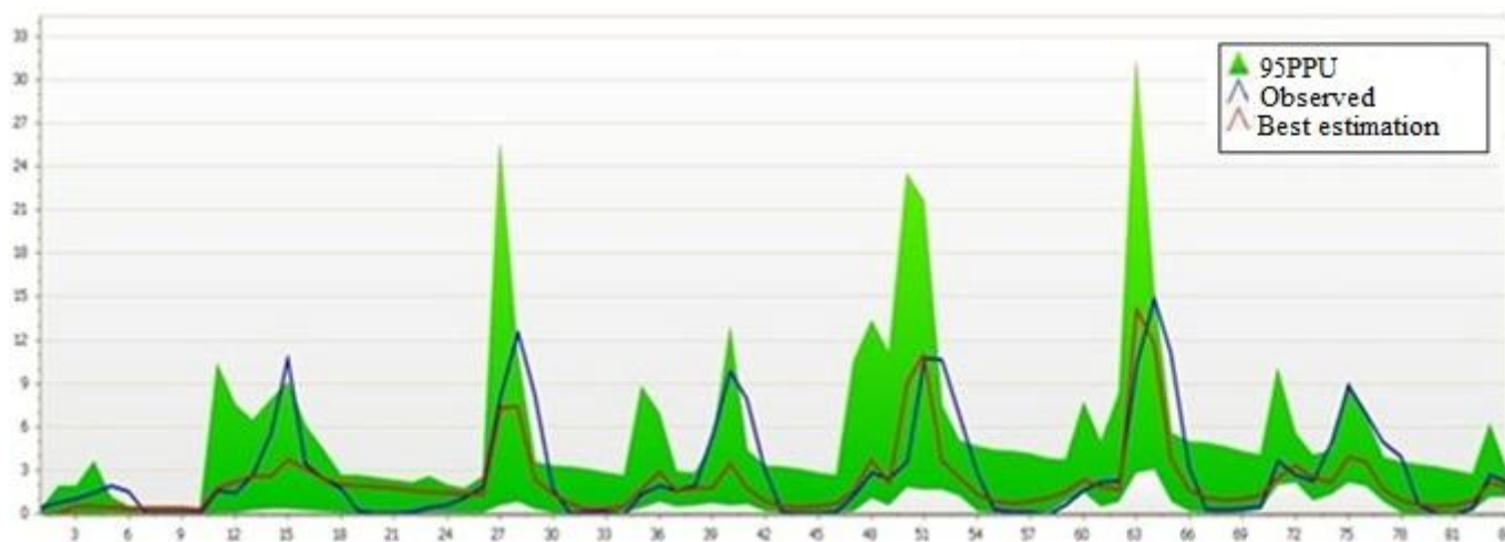
شکل ۴- نمودار عدم قطعیت در دوره واسنجی Fig 4. Diagram of uncertainty in the calibration period
