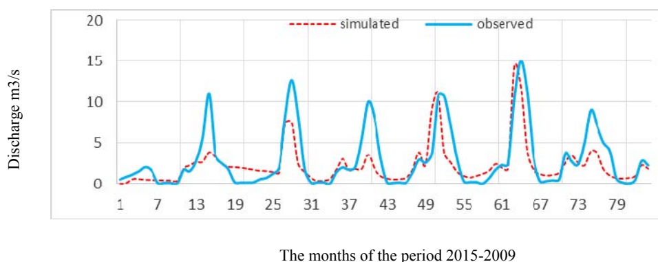
شکل ۶- مقایسه هیدروگراف های شبیه سازی شده و مشاهداتی در دوره اعتبارسنجی با پایه زمانی ماهانه.
