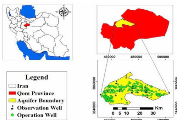
شکل ۱- نقشه موقعیت منطقه مطالعه در ایران و استان قم Fig 1. Location map of the study area in Iran and Qom province
