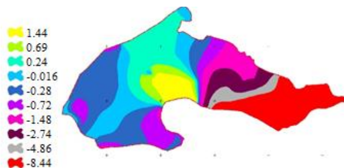
شکل ۷- تغییرات تراز سطح آب در سال‌های ۱۳۷۶(الف)، ۱۳۷۷(ب)، ۱۳۷۸(ج)، ۱۳۷۹(د) و ۱۳۸۰(ه) نسبت به سال ۱۳۷۱ Fig 7. Water level changes in the years 1997(a), 1998(b), 1999(c), 2000(d) and 2001(e) compared to 1992
