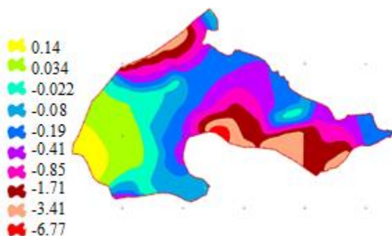
شکل ۷- تغییرات تراز سطح آب در سال‌های ۱۳۷۶(الف)، ۱۳۷۷(ب)، ۱۳۷۸(ج)، ۱۳۷۹(د) و ۱۳۸۰(ه) نسبت به سال ۱۳۷۱ Fig 7. Water level changes in the years 1997(a), 1998(b), 1999(c), 2000(d) and 2001(e) compared to 1992
