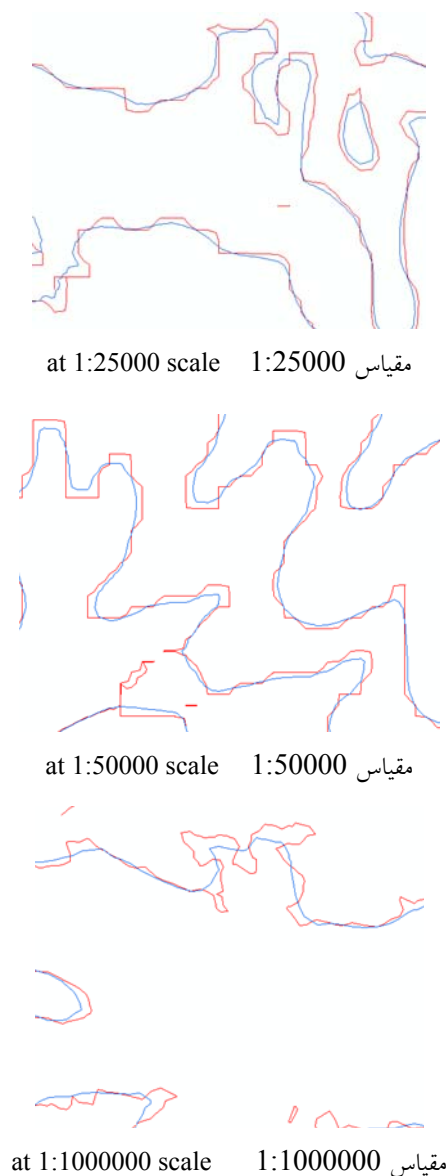
شکل ۱۰- اثر الگوریتم‌های چندمقیاسی در ساده‌سازی داده‌های ارتفاعی (خطوط قرمز: قبل از ساده‌سازی و خطوط آبی: پس از ساده‌سازی)
