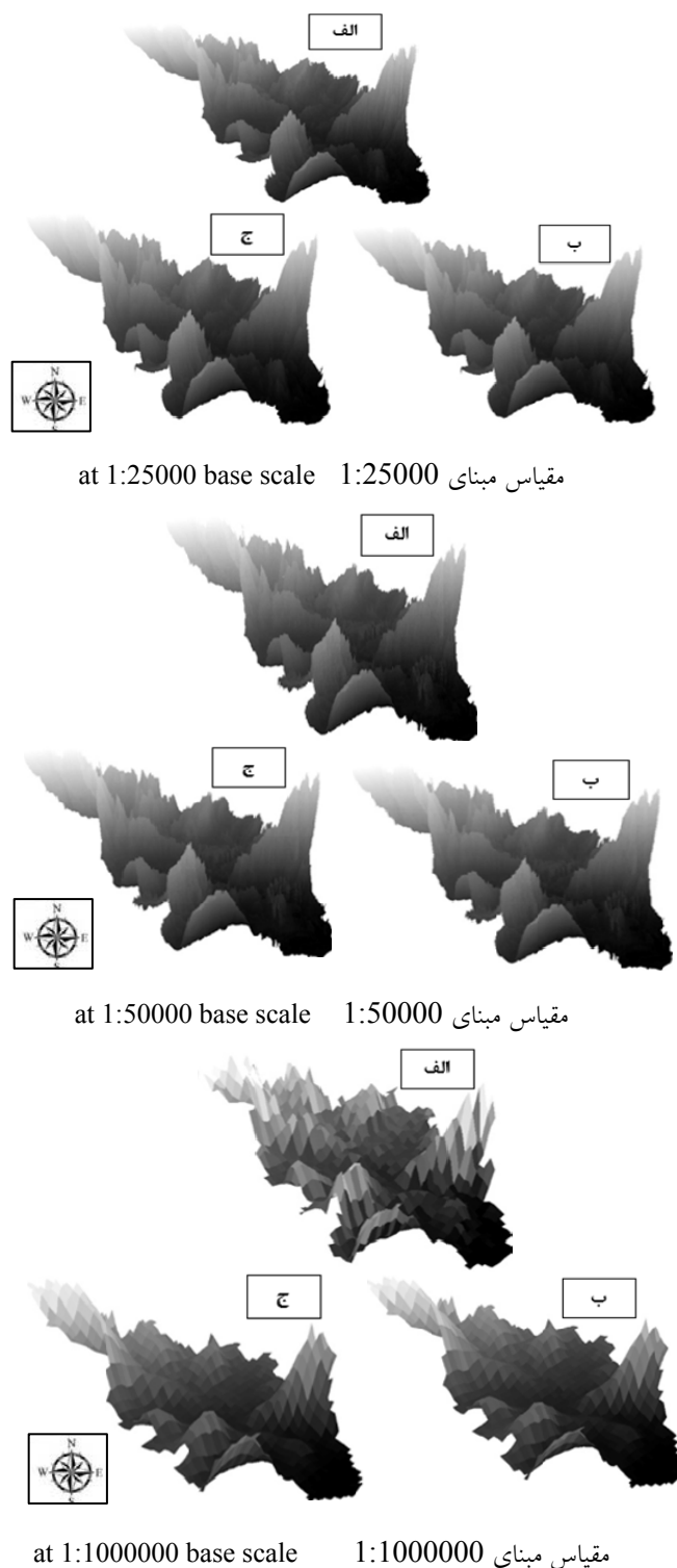
الف- قبل ساده‌سازی ب- فیلتر پایین‌گذر ج- میانگین ساده a) Before simplification b) low pass filter c) simple average
