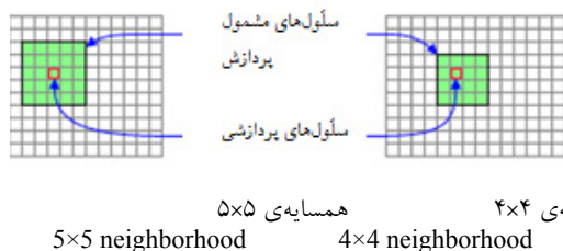
شکل ۷- محاسبه‌ی توابع آماری با همسایه‌ی مستطیلی شکل [۳]
