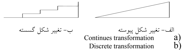
شکل ۳- انواع تغییر شکل‌ها در نمایش چندمقیاسی [۱۸]
