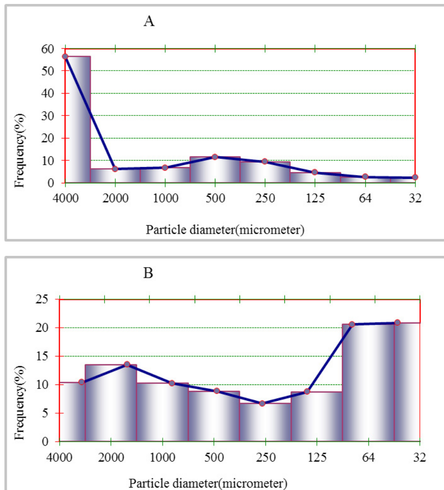
شکل ۶- هیستوگرام و منحنی‌های دانه‌بندی - A عرصه شاهد و B بند علویه
