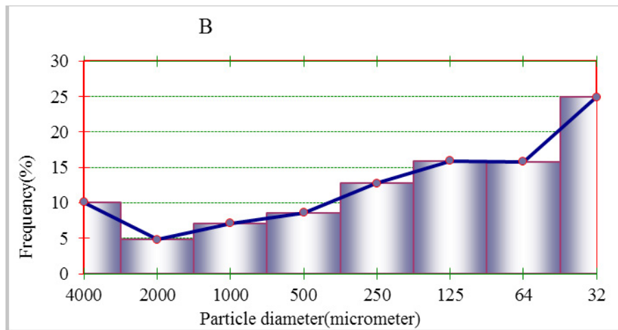
شکل ۸- هیستوگرام و منحنی‌های دانه‌بندی - A عرصه شاهد B بند صدرآباد
