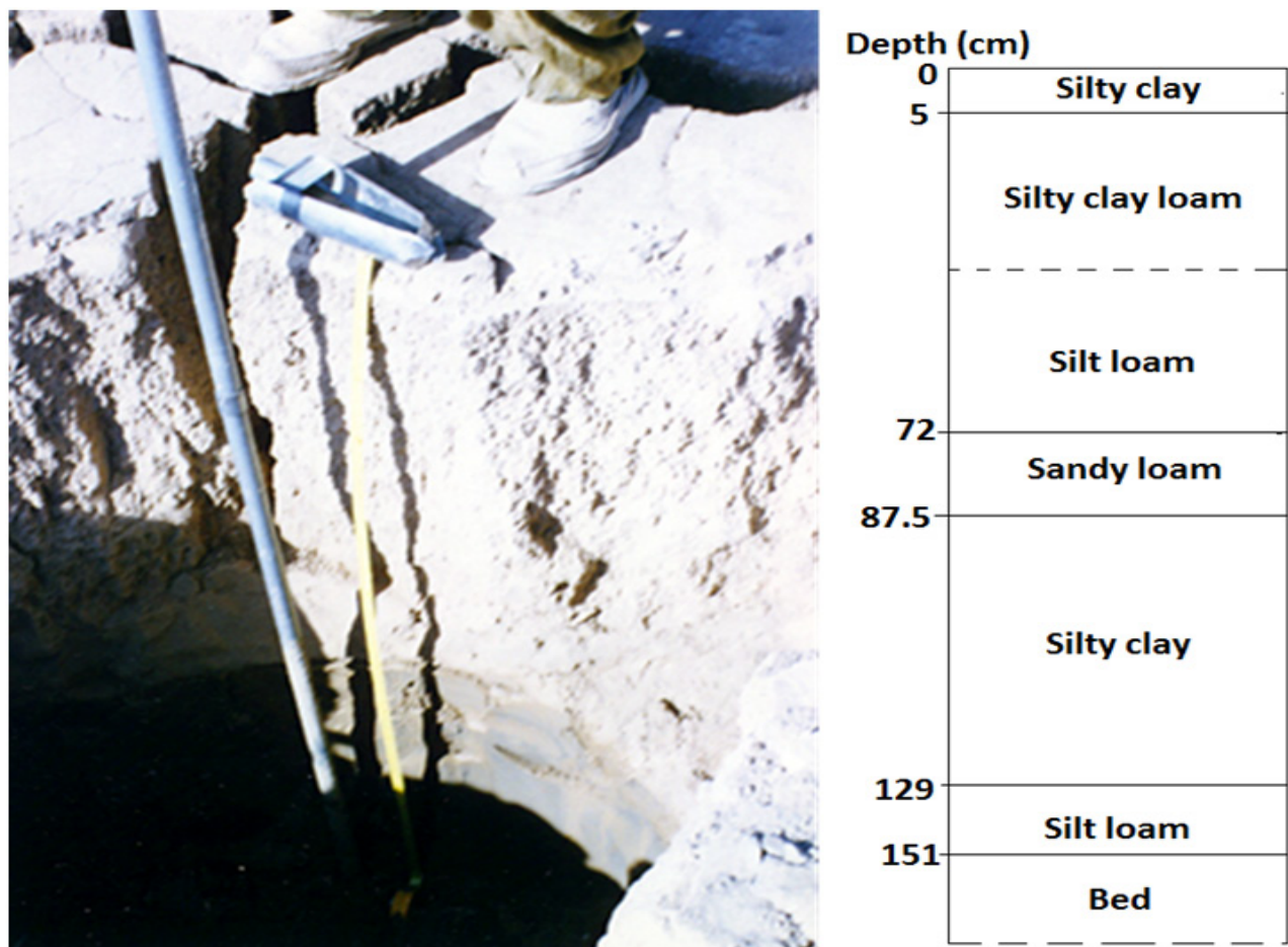
شکل ۵- یک نیمرخ نمونه در رسوبات دریاچه‌ای مربوط به خشک‌رود چمرود (تصویر چپ) و تفاوت بافت در لایه‌های مختلف (تصویر راست) [۶]
