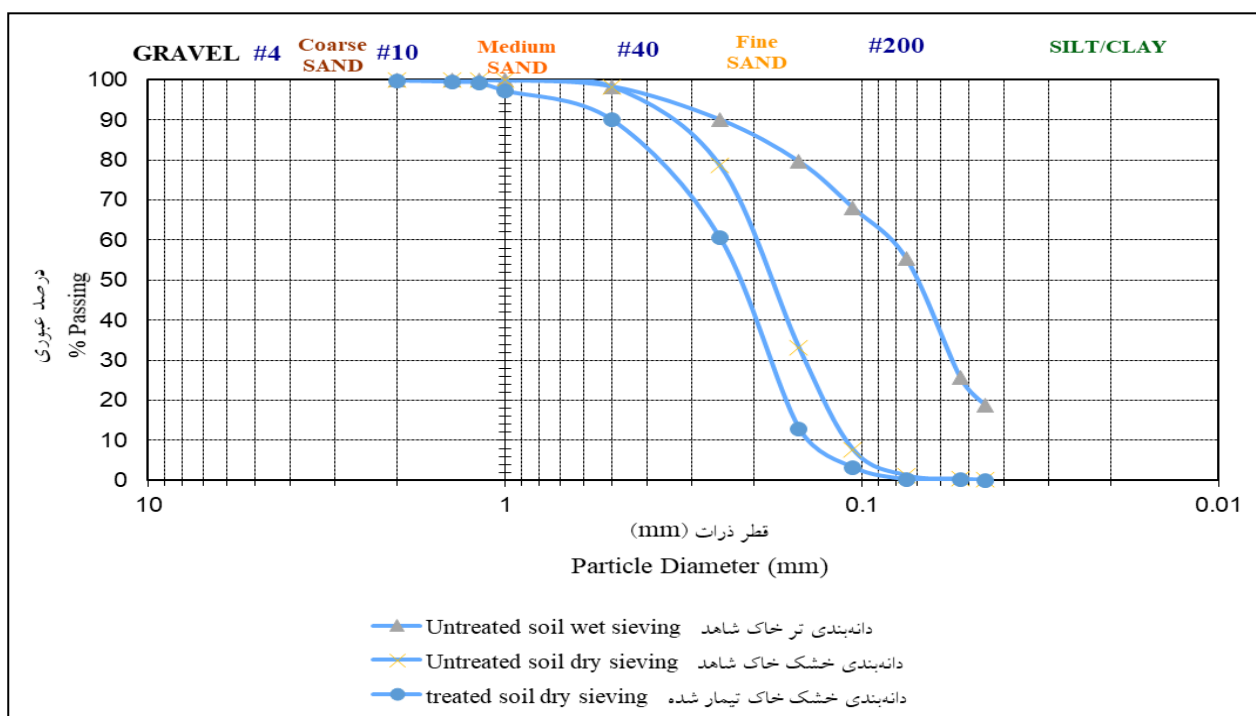
شکل ۷- نمودار دانه بندی خاک شاهد و خاک تیمار شده با ۱/۲ گرم بر مترمربع گوار Fig 7. Sieve analysis data for untreated soil and soil treated with 1.2 gr/m 2 Guar
