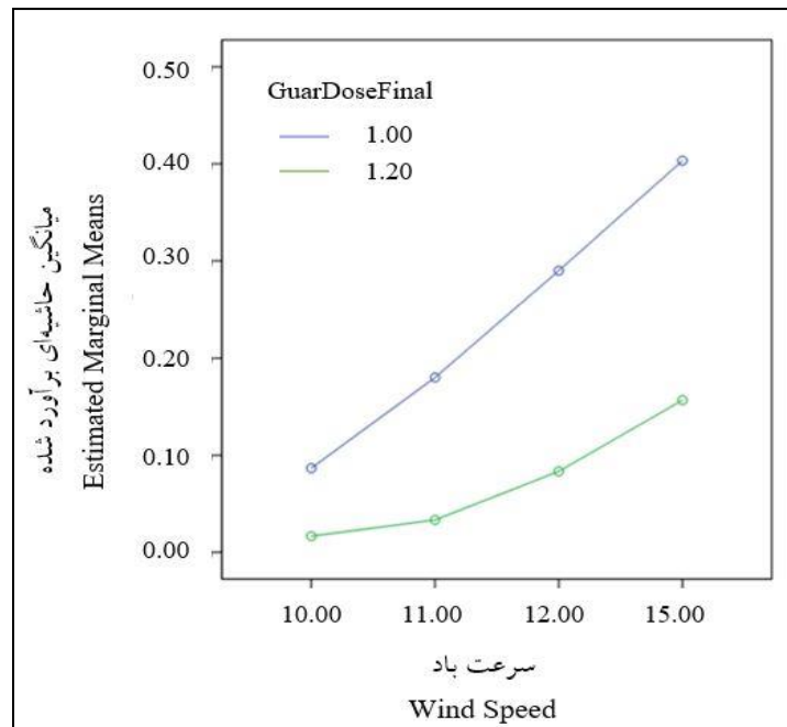
شکل ۶- برآورد میانگین حاشیه‌ای فرسایش Fig 6. Estimated marginal means of erosion
