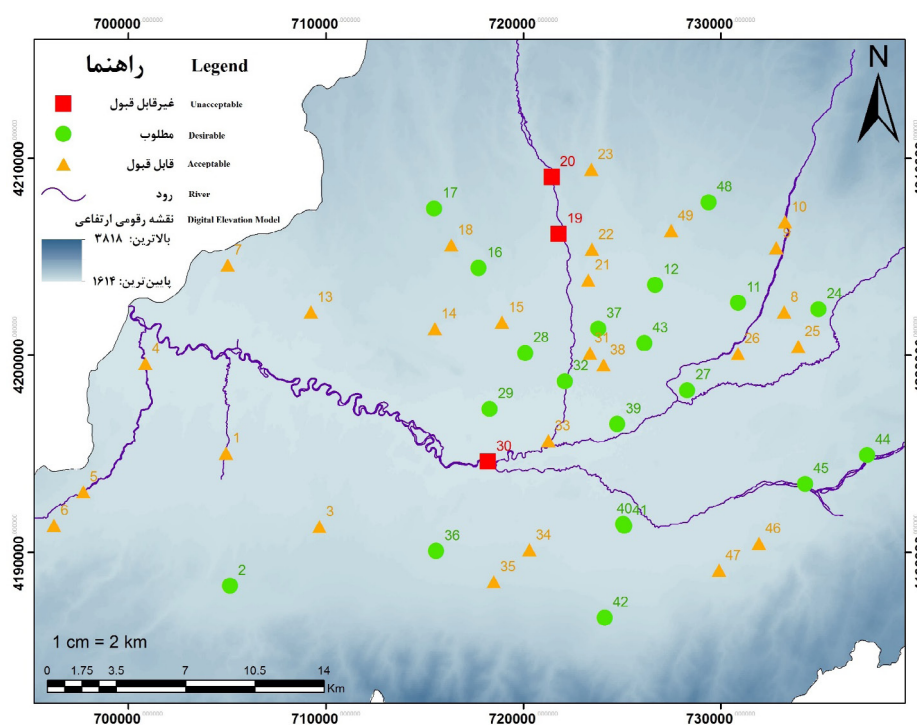
شکل ۵- تغییرات مکانی کیفیت آب زیرزمینی دشت سراب
