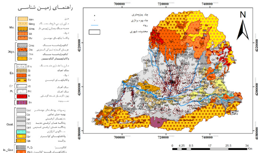
شکل ۱- نقشه زمین‌شناسی و موقعیت جغرافیایی دشت سراب. Fig 1. Geology and Geographical situation of Sarab plain
