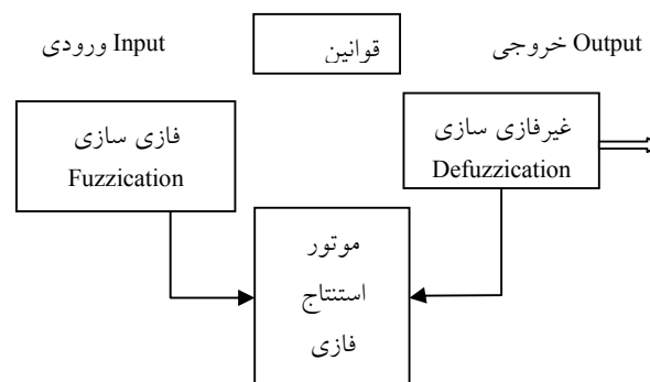
شکل ۲- سیستم استنتاج فازی [۲۵].
