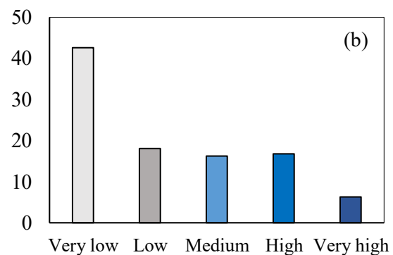
شکل ۳-الف: نقشه پیش‌بینی مکانی پتانسیل چشمه‌های آب زیرزمینی ب: فراوانی نسبی کلاس‌های استعداد پیش‌بینی مکانی پتانسیل چشمه آب زیرزمینی.
