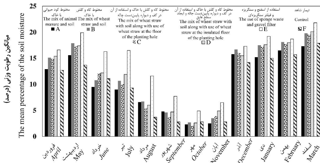
شکل ۵- میانگین رطوبت تیمارهای مختلف سامانه‌های سطوح آبگیر باران در ماه‌های مختلف سال
