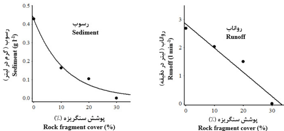
شکل ۳- تاثیر پوشش سنگریزه در جریان سطحی ۷/۵ لیتر در دقیقه بر میزان رواناب و رسوب Fig. 3. Effect gravel cover in surface flow 7.5 L min -1 on runoff and sediment
