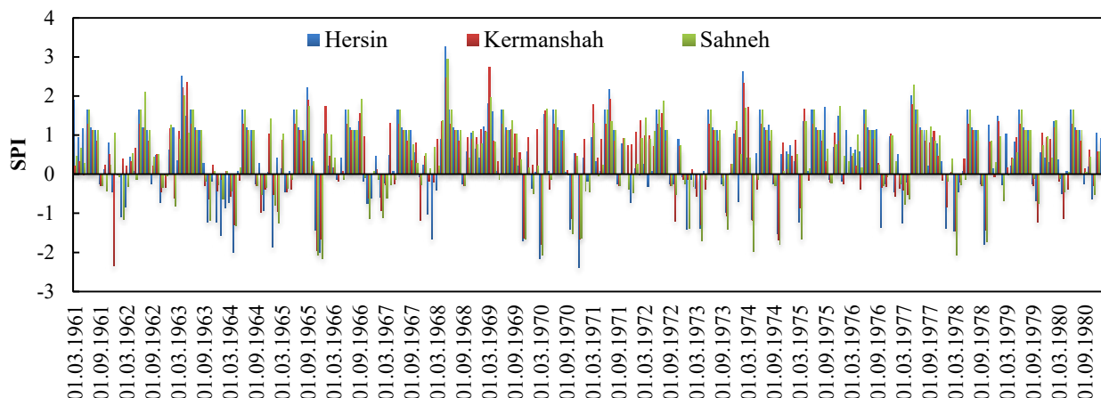
شکل ۲- مقادیر شاخص خشک‌سالی SPI ماهانه در دوره ۱۳۵۹-۱۳۴۰ در استان کرمانشاه
