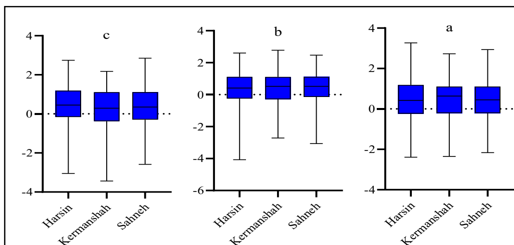
شکل ۵- توزیع شاخص خشک سالی SPI ماهانه طی ۱۳۴۰ تا ۱۳۹۹ ایستگاه‌های مختلف در استان کرمانشاه برای دوره‌های ۱۳۵۹(a)-۱۳۴۰، ۱۳۷۹(b)-۱۳۶۰ و ۱۳۹۹(c)-۱۳۸۰
