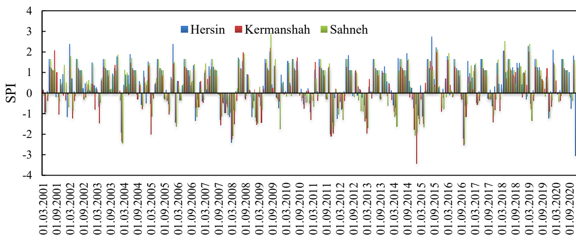
شکل ۴- مقادیر شاخص خشک‌سالی SPI ماهانه در دوره ۱۳۹۹-۱۳۸۰ در استان کرمانشاه
