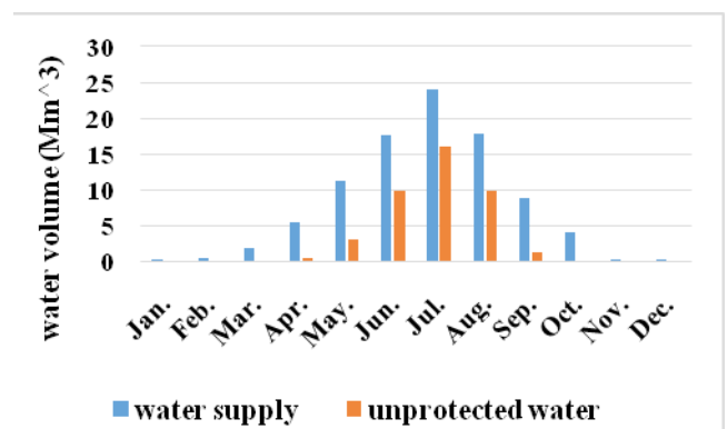
شکل ۷- حجم نیاز آبی و آب تأمین نشده (میلیون مترمکعب) در سناریوی واقع‌گرایانه
