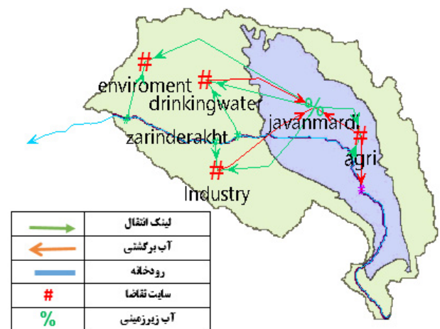
شکل ۳- شماتیک مدل تخصیص آب در حوزه آبخیز خانمیرزا در محیط WEAP
