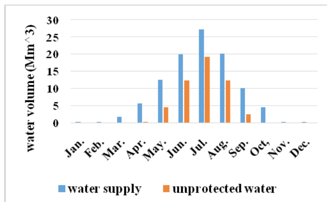
شکل ۴- حجم نیاز آبی و آب تأمین نشده (میلیون مترمکعب) در سناریوی مرجع
